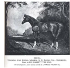
Algol 1928
